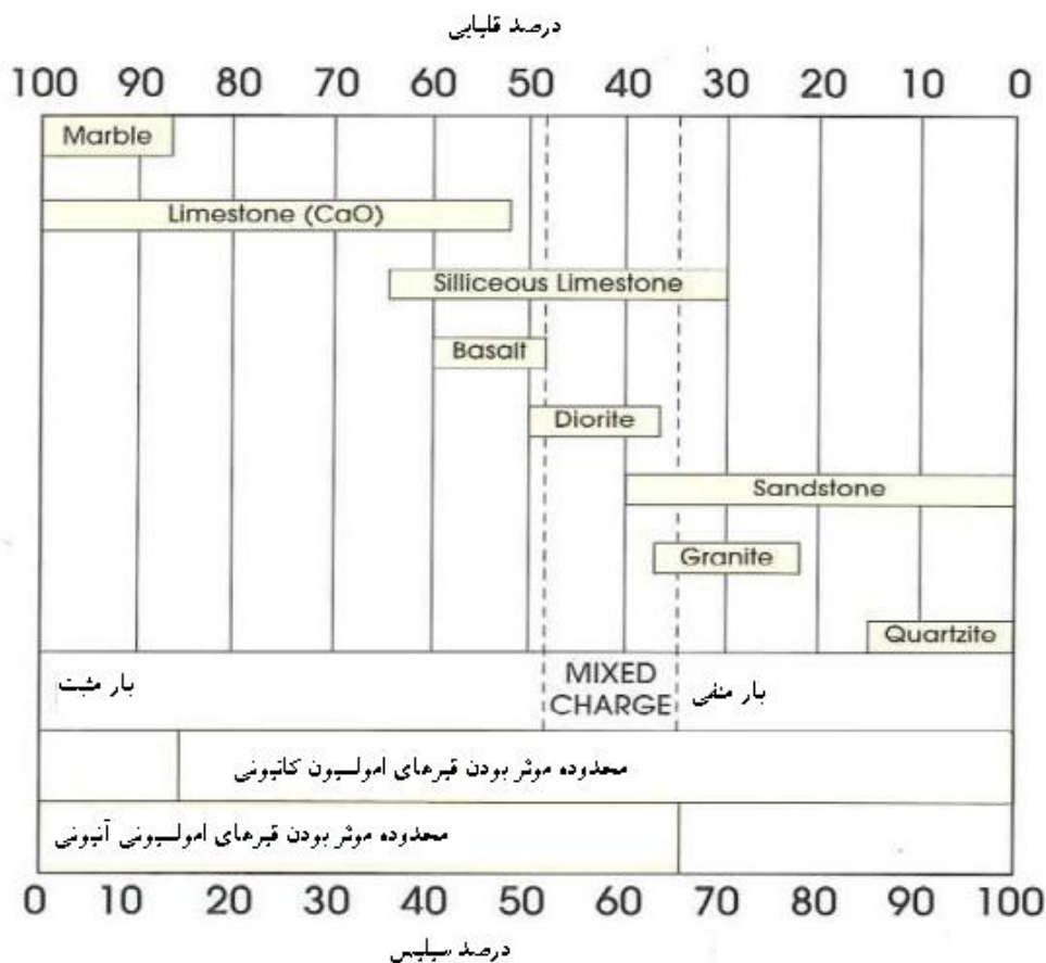
شکل ۱-۲ راهنمای انتخاب نوع قیر امولسیون بر اساس جنس مصالح سنگی
