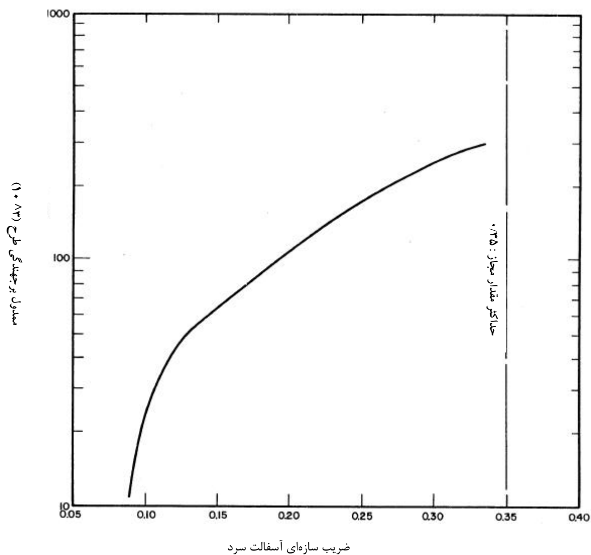
شکل ۴-۲ ارتباط بین پارامتر مدول برجهندگی و عدد استحکام مارشال در ۲۲ درجه سانتیگراد [۵]
