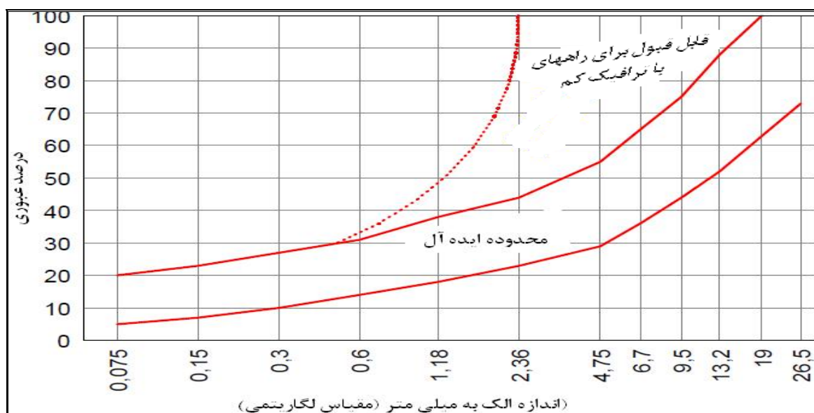
شکل ۱- حدود دانه بندی پیشنهادی برای تهیه آسفالت سرد کفیری
