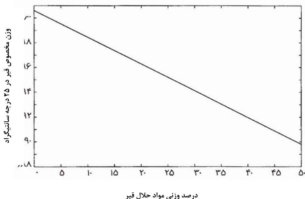
شکل ۱-۳ تغییرات وزن مخصوص یک نمونه قیر در ۲۵ درجه سانتیگراد بر حسب میزان مواد حلال آن
