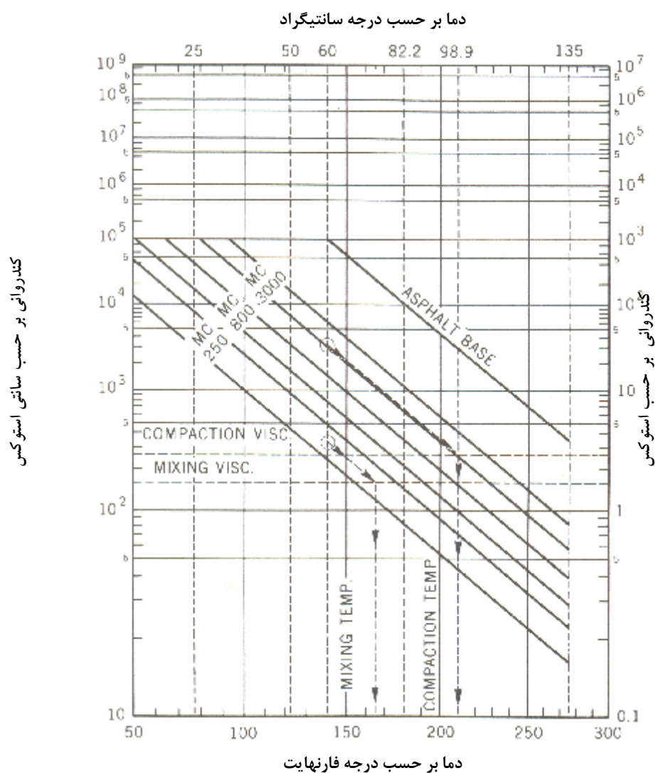
شکل ۳-۲- دمای اختلاط باتوجه به نمودار دما- کندروانی
