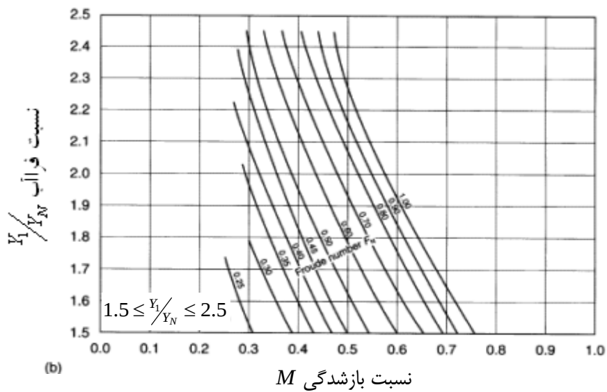
شکل ۱۰- منحنی تغییرات Y_1/Y_N در مقابل نسبت بازشدگی M و عدد فرود عمق نرمال Fr_N
