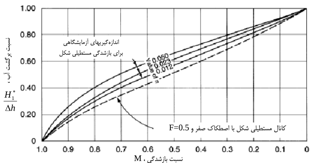
شکل ۶- نسبت برگشت آب در روش USGS برای شرایط اولیه در تستهای آزمایشگاهی (وجود بازدهی با کوله‌های قائم و لبه‌های ورودی تیز و بدون گردگوشی)
