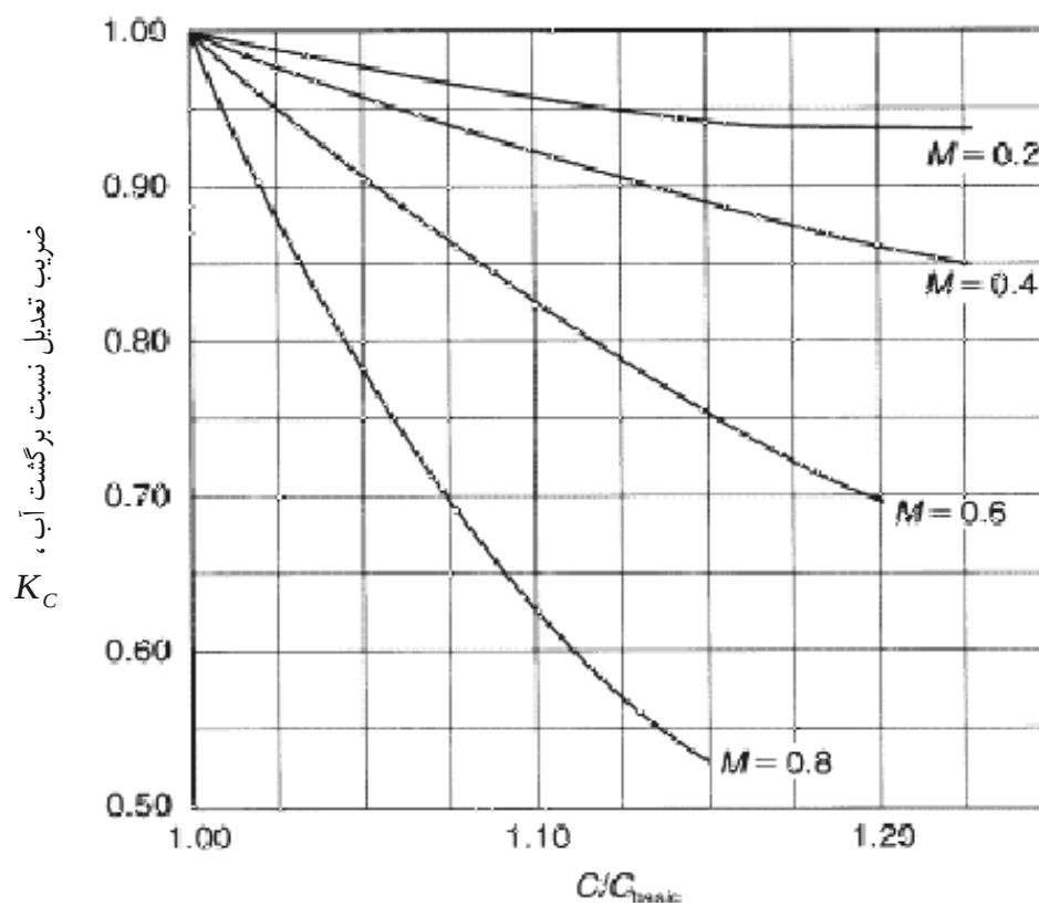
شکل ۷- تعیین ضریب K_c در روش USGS
