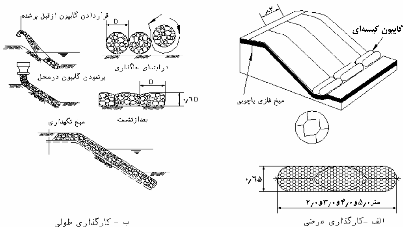
شکل ۳۲- کاربرد و مشخصات گابیون کیسه‌ای
