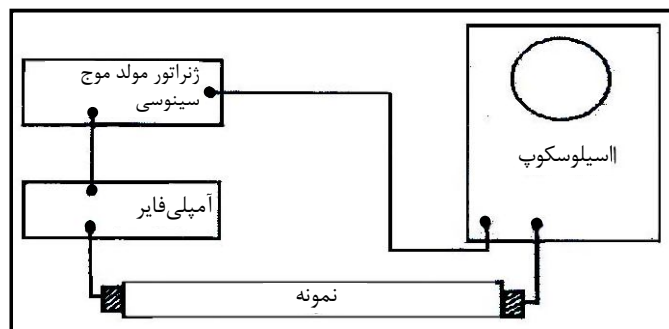
شکل ۷-۱- نحوه قرارگیری فرستنده و گیرنده روی نمونه در آزمایش بسامد تشدید
