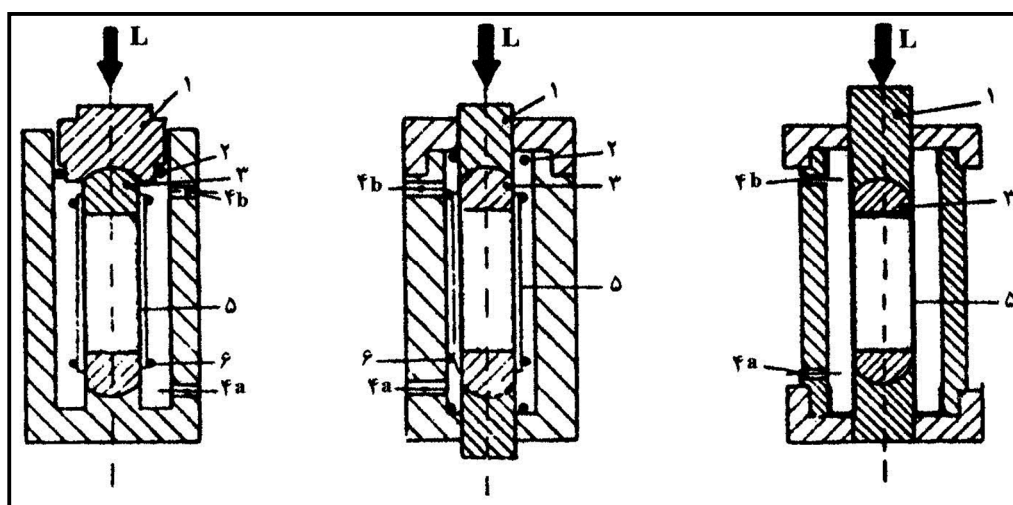
شکل ۲-۱۷- سه نوع مختلف از محفظه سه محوری و اجزای آن‌ها
