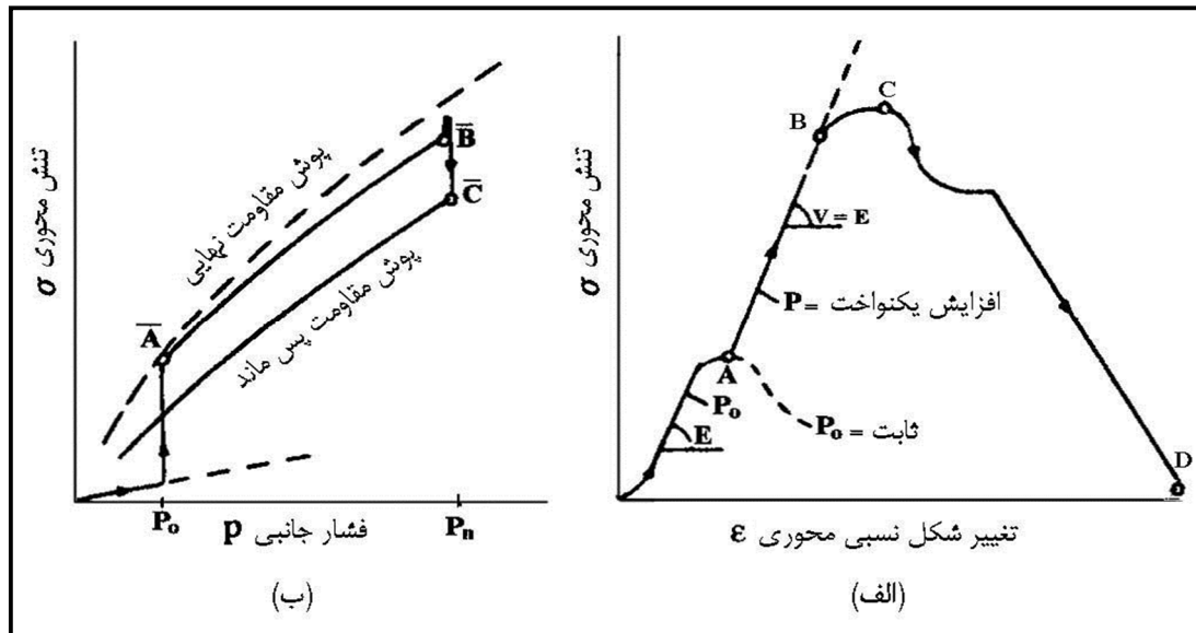
شکل ۲-۲۰- نمودار شماتیک نتیجه آزمایش به روش ج (شکست پیوسته)
