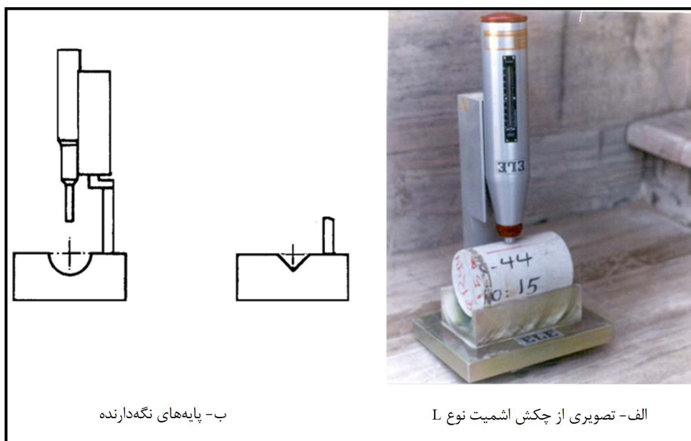
شکل ۲-۱۱- تصویری از چکش اشمیت نوع L و پایه‌های نگه‌دارنده
