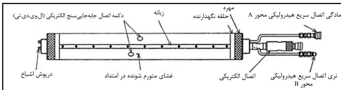
شکل ۳-۱۱- دیلاتومتر نوع لنک
