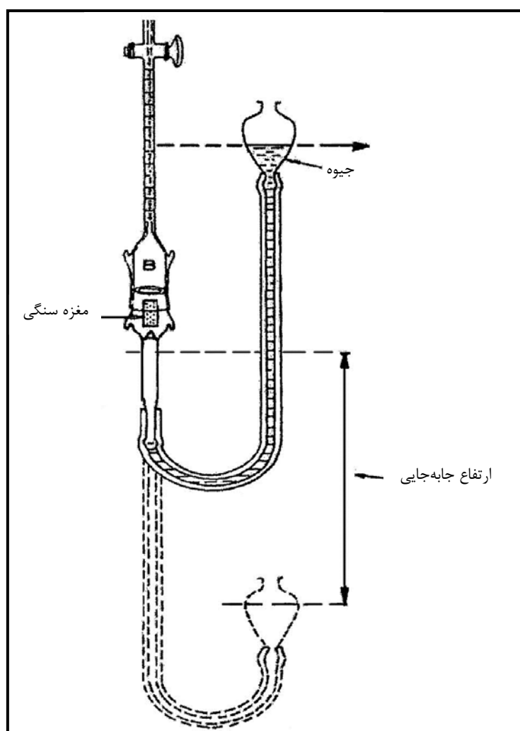
شکل ۱-۱- دستگاه تخلخل‌سنج با روش جابه‌جایی جیوه، نوع واشبرن - بونتینگ ۱
