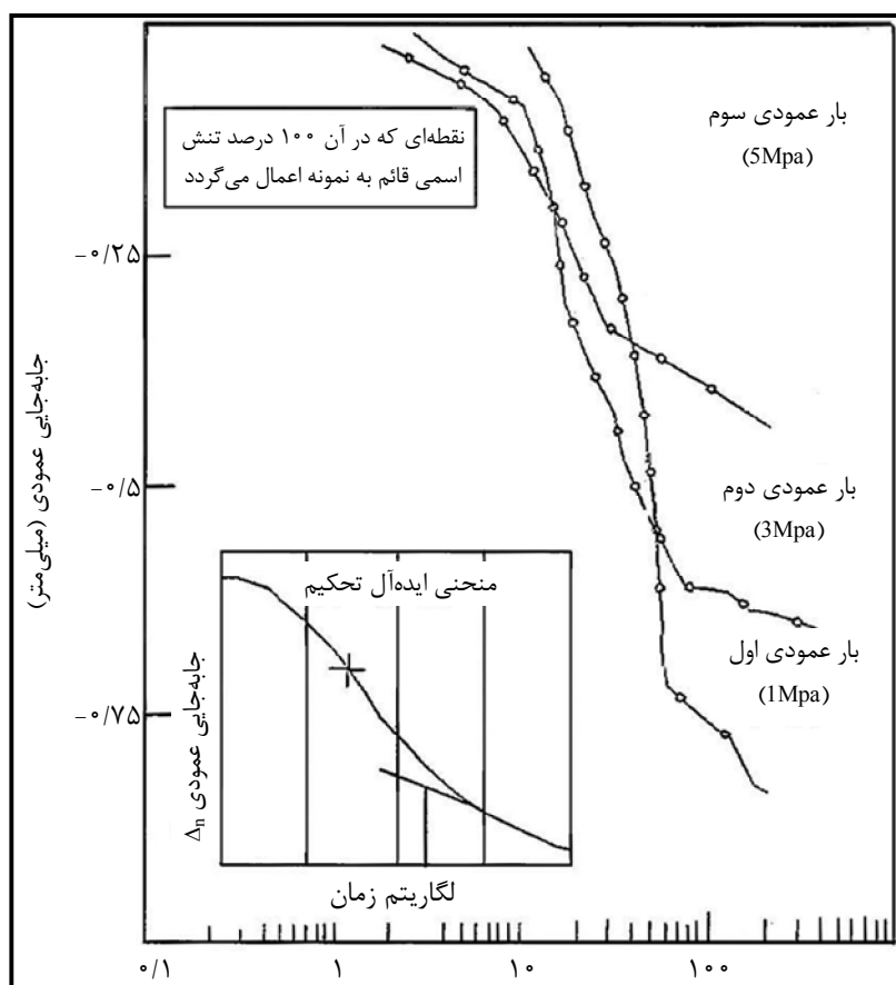
شکل ۳-۲۳- منحنی تحکیم بار عمودی
