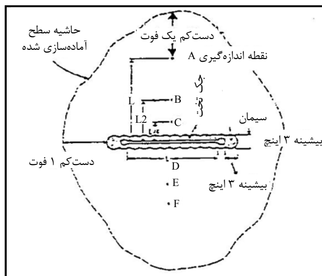
شکل ۳-۱۳- آرایش تجهیزات اندازه‌گیری جک مسطح در اطراف شکاف
