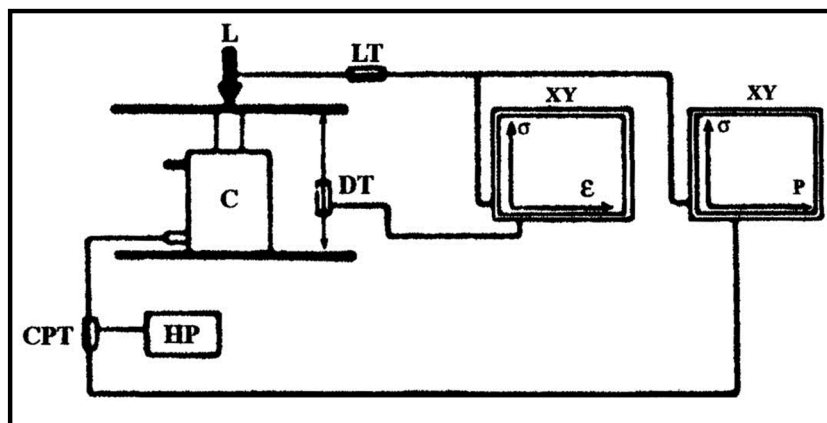
شکل ۲-۱۸- شمای ساده دستگاه آزمایش سه محوری
