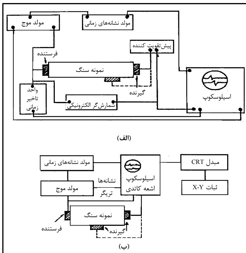
شکل ۱-۴- دو نوع مدار مختلف برای انجام آزمایش
