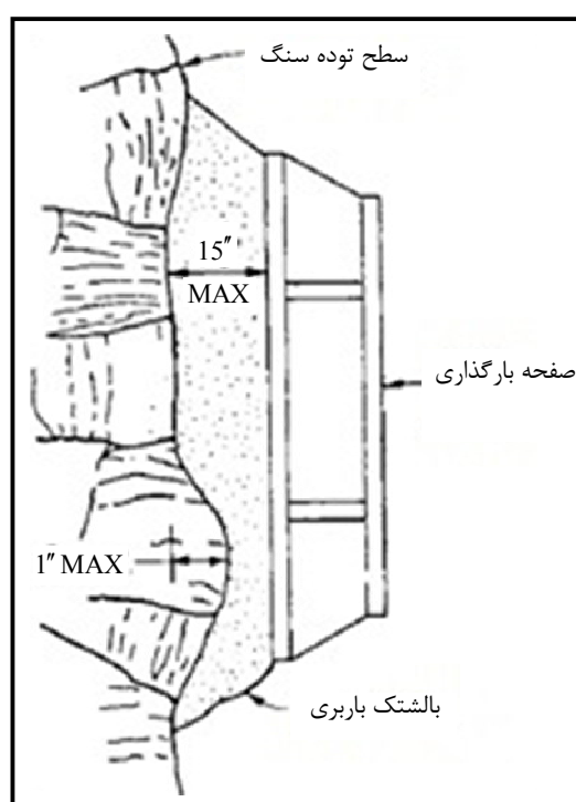
شکل ۳-۸- ابعاد مجاز سطح سنگ و بالشتک بتنی
