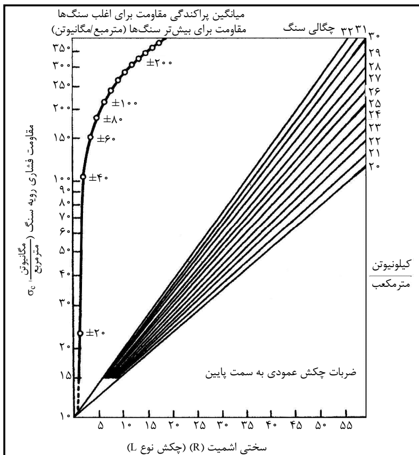
شکل ۲-۱۳- نمودار وابستگی مقاومت فشاری سنگ به عنوان تابعی از شمار سختی واجهشی اشمیت و چگالی خشک
