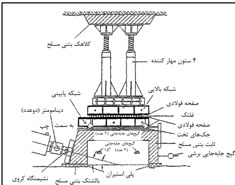
شکل ۳-۲۱- نمایش تجهیزات مورد نیاز بر حسب محل قرارگیری در آزمایش برش برجا
