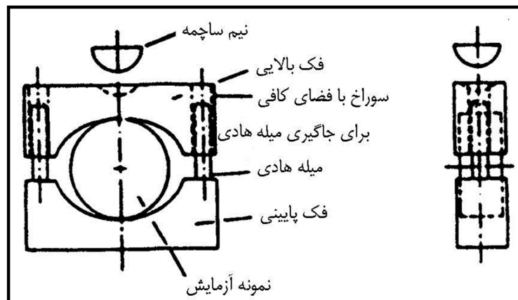
شکل ۲-۳- ابزار آزمایش برزلی
