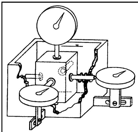
شکل ۲-۱۵- سلول و نمونه آماده شده برای انجام آزمایش آماسی نامحصور
