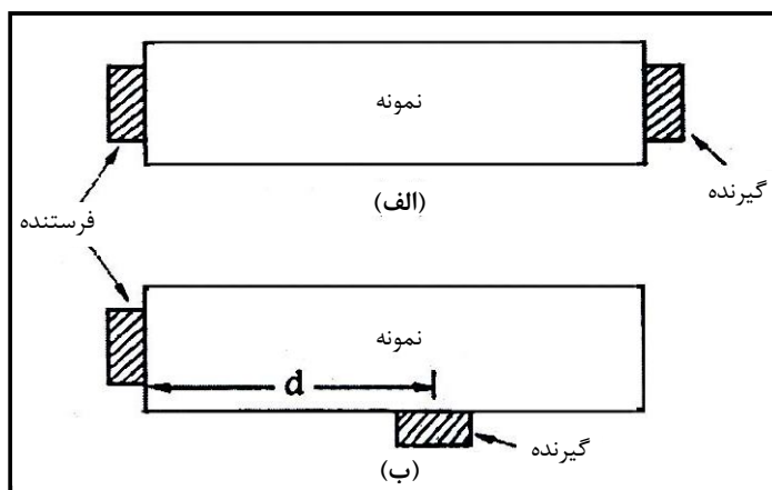
شکل ۱-۵- نحوه قرارگیری فرستنده و گیرنده روی نمونه در آزمایش با موج بسامد بالا الف- روش انتشار موج ب- روش مقطع لرزه‌ای
