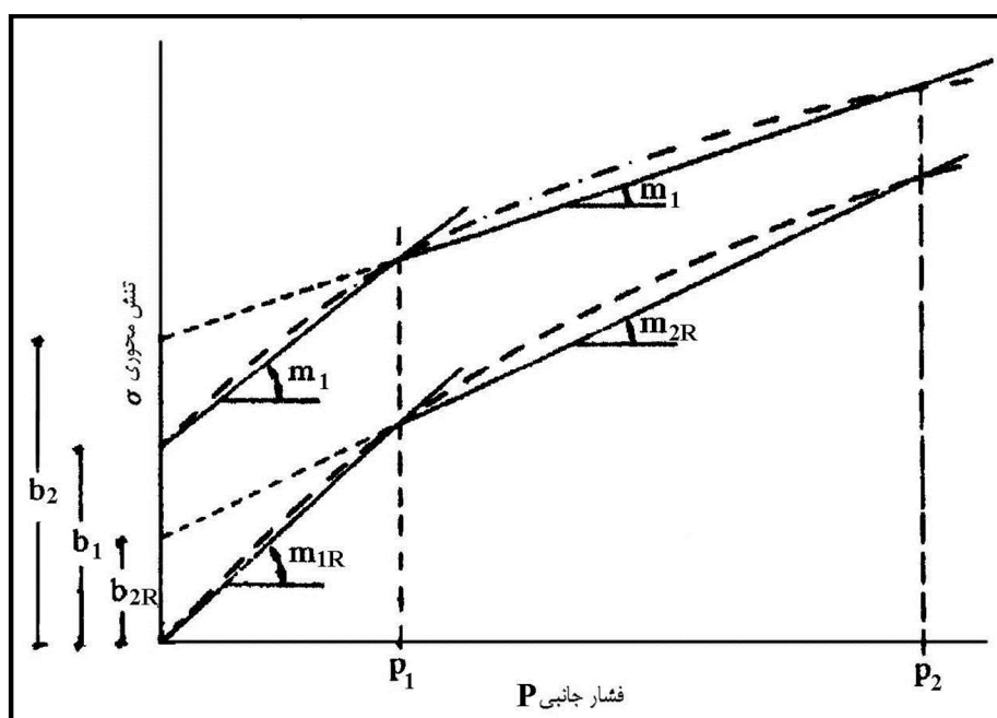
شکل ۲-۲۱- نمودار شماتیک پوش‌های مقاومت نهایی و پسماند
