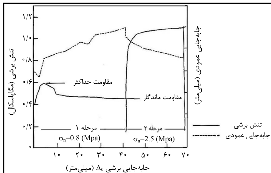
شکل ۳-۲۴- منحنی تنش برشی - جابه‌جایی برشی و جابه‌جایی عمودی - جابه‌جایی برشی در آزمایش برش برجا
