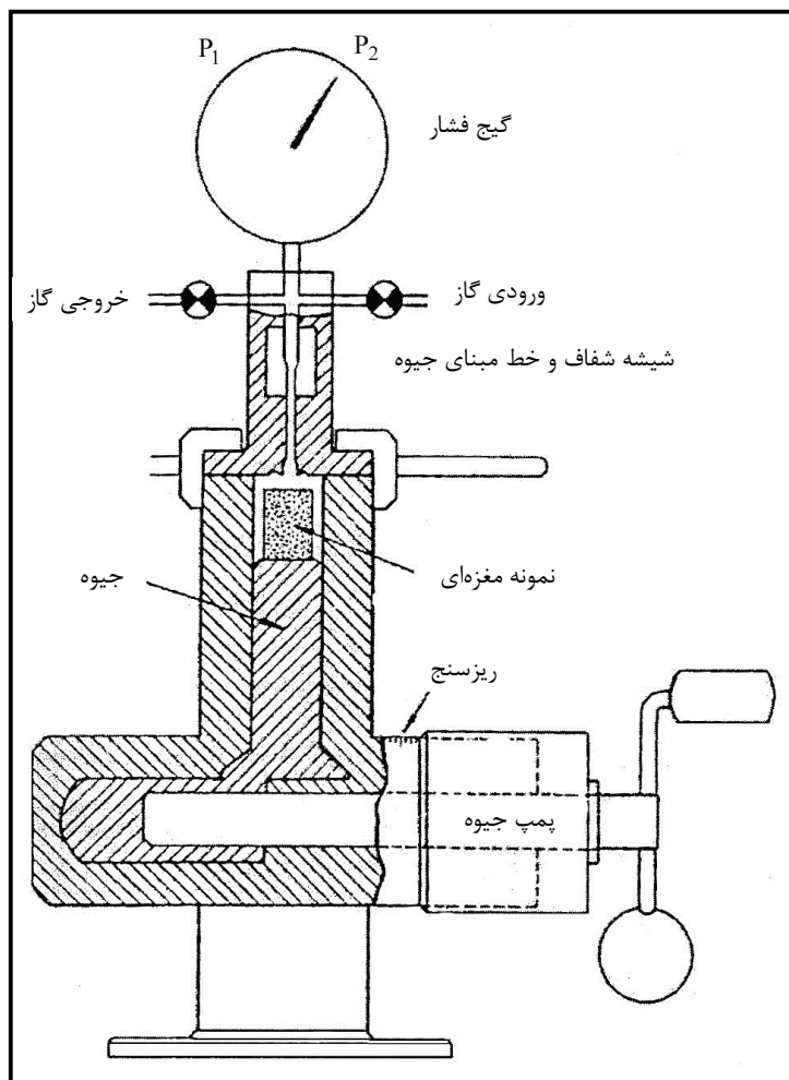
شکل ۱-۲- نمایش شماتیک از تخلخل سنج قانون بویل، نوع کوبه
