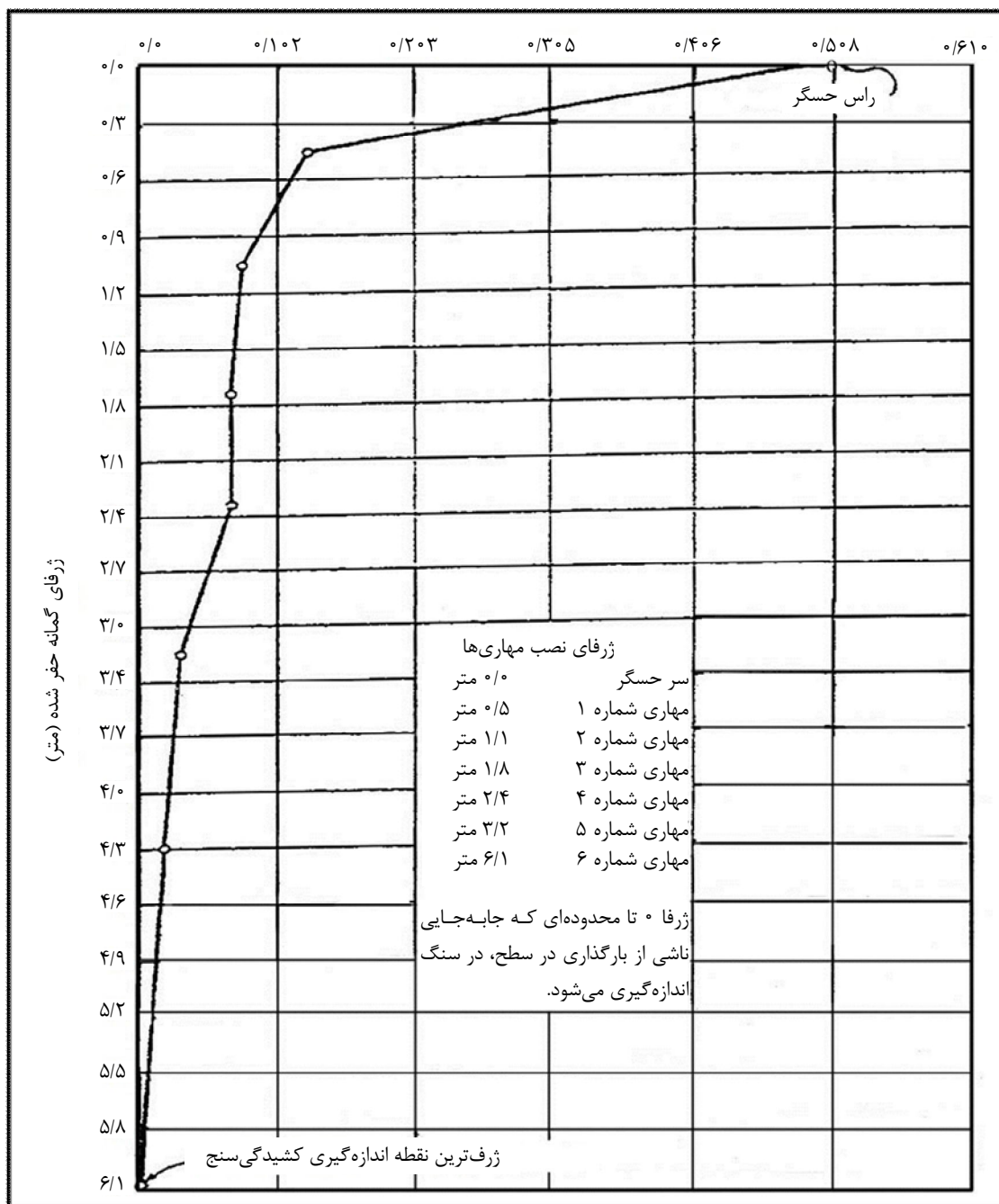
شکل ۳-۵- جابه‌جایی محوری بر حسب زرفا، نسبت به زرف‌ترین نقطه درگیر، زیر فشار ۶/۹ مگاپاسکال
