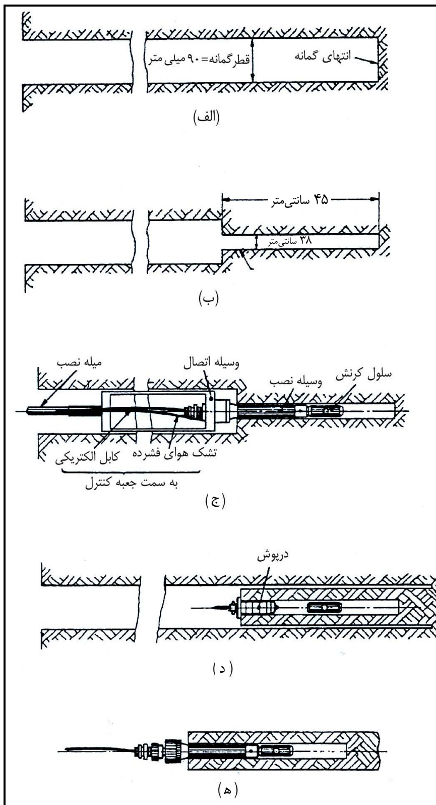
شکل ۳-۲۰- مراحل مختلف انجام آزمایش مغزه‌گیری محیطی الف- حفاری گمانه تا ژرفای مورد نظر، ب- حفاری چال ۳۸ میلی‌متر، ج- نصب محفظه کرنش‌سنج، د- نصب درپوش و ه- مغزه آزاد شده از گمانه
