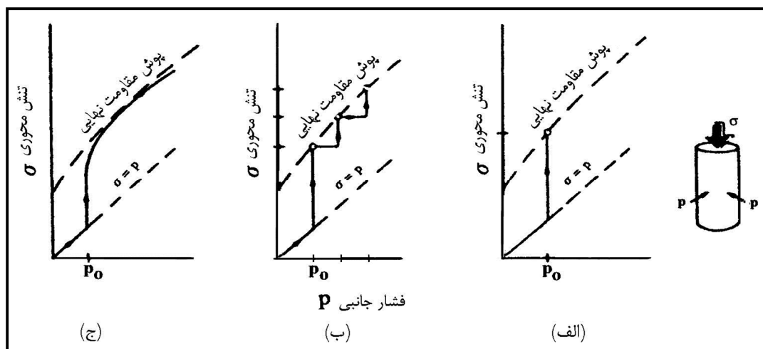
شکل ۱۶-۲- روش‌های مختلف آزمایش مقاومت فشاری سه محوری سنگ
