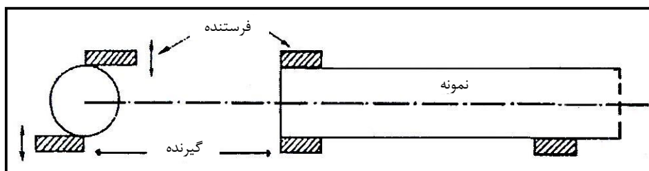
شکل ۶-۱- نحوه قرارگیری فرستنده و گیرنده روی نمونه در آزمایش با موج فرکانس پایین
