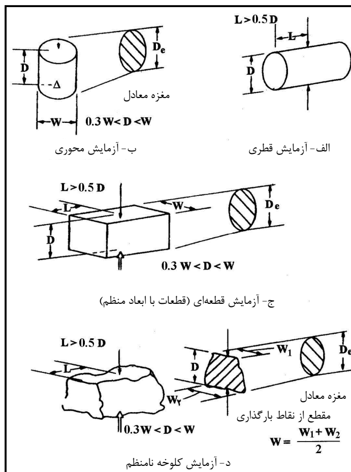
شکل ۲-۶- شرایط هندسی نمونه‌ها در آزمایش بار نقطه‌ای
