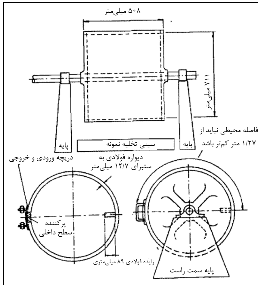
شکل ۱-۳- نمایش شماتیک دستگاه لس آنجلس
