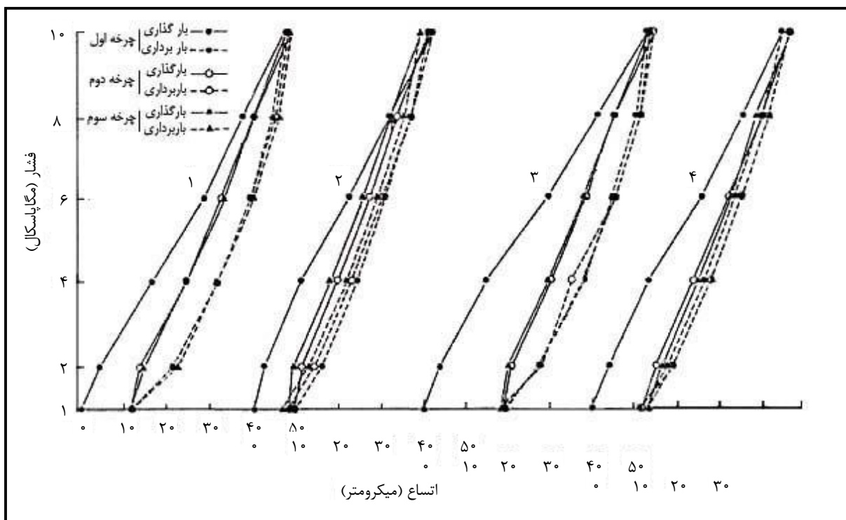
شکل ۳-۱۲- منحنی‌های فشار در مقابل اتساع مربوط به چهار سنجش‌گر نصب شده در یک اتساع سنج لنک
