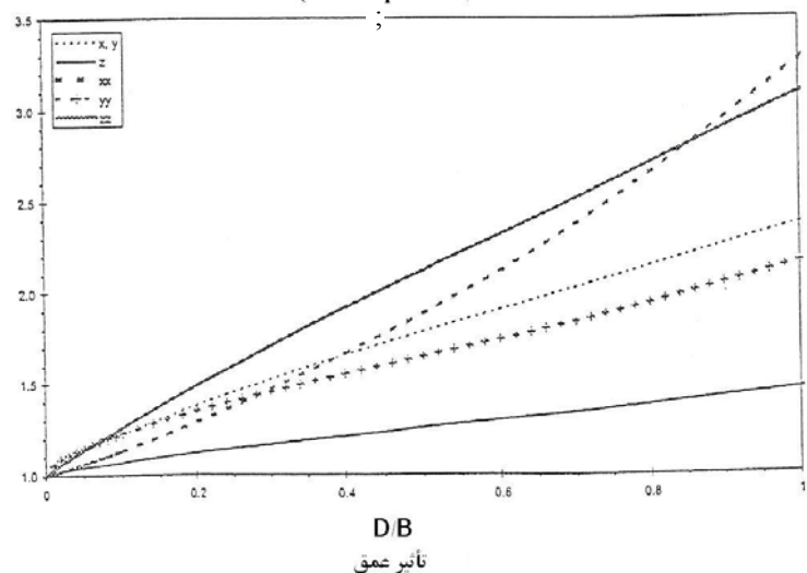
شکل (ت ۳-۴): اثرات شکل و عمق شالوده
