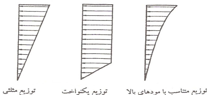
شکل (ت ۳-۶) - حالت‌های مختلف توزیع نیروی جانبی
