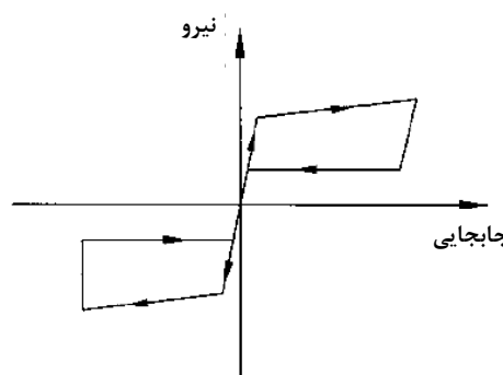
وسیله اصطکاکی-فنری با قابلیت تامین
