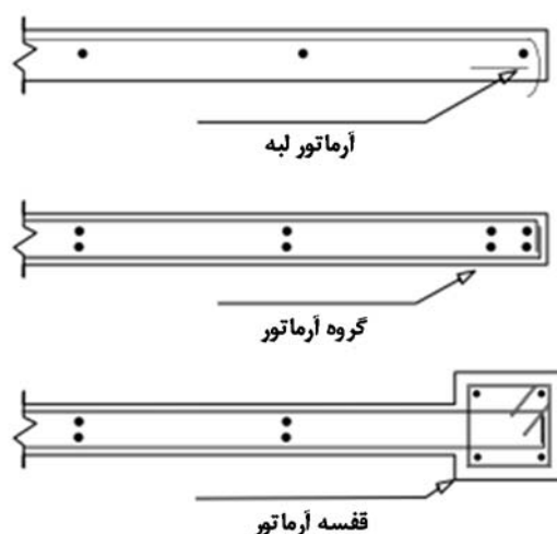
شکل ت ۱۱-۱۱: آرماتور گذاری دیوار برشی
