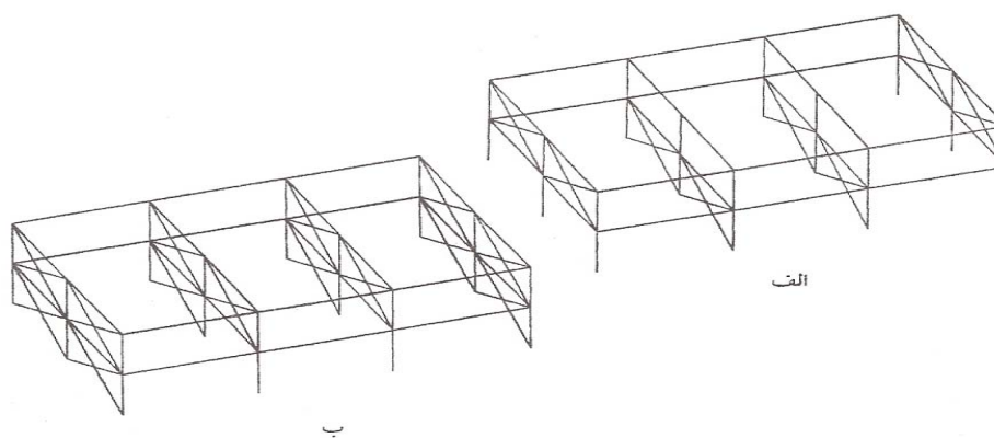
شکل (ت ۳-۸) - دو سیستم سازه ای که در آنها دیافراگم در مسیر انتقال بار جانبی قرار گرفته است.
