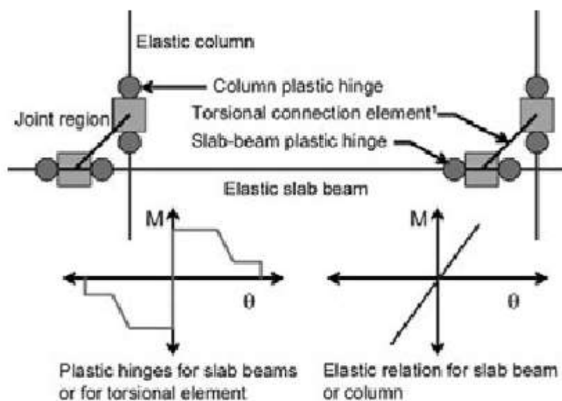
شکل ت (۶-۱): مدلسازی اتصال دال-ستون
