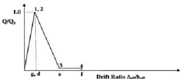
شکل ت-۷-۲- رابطه نیرو- تغییر شکل اعضای نیرو کنترل
