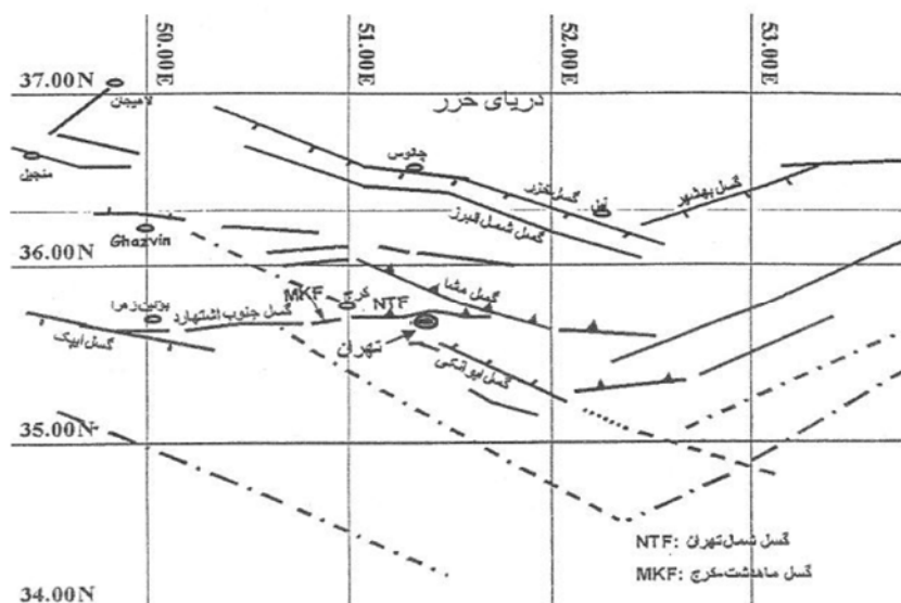
شکل (ت ۱-۳): گسله‌های بنیادی ناحیه تهران
