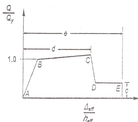
شکل (۸-۸): رابطه ی کلی نیرو - تغییر مکان برای دیوارهای مصالح بنایی
