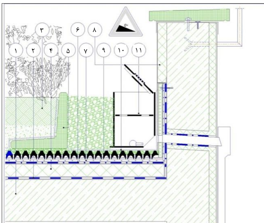
شکل ۲-۵- مقطع بام سبز نیمه فشرده، مأخذ: شرکت دیادم
